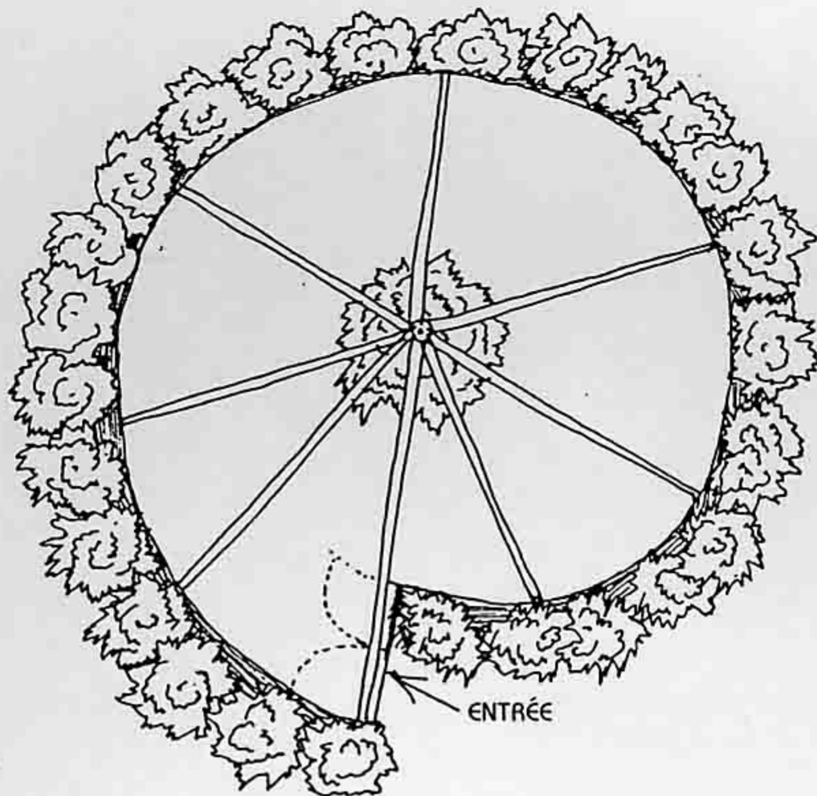
FIG. 6.9 : « MAISON DE PLANTES » 1 (PLAN) DALLE DE BÉTON AU SOL, SPIRALE DE BAMBOU OU DE PEUPLIER, PILIER CENTRAL CONSTITUÉ PAR UN ARBRE EXISTANT. LES MURS SONT TISSÉS ET COUVERTS DE LIERRE JUSQU'AU TOIT. C'EST UN ABRI BON MARCHÉ POUR LE BÉTAIL.
