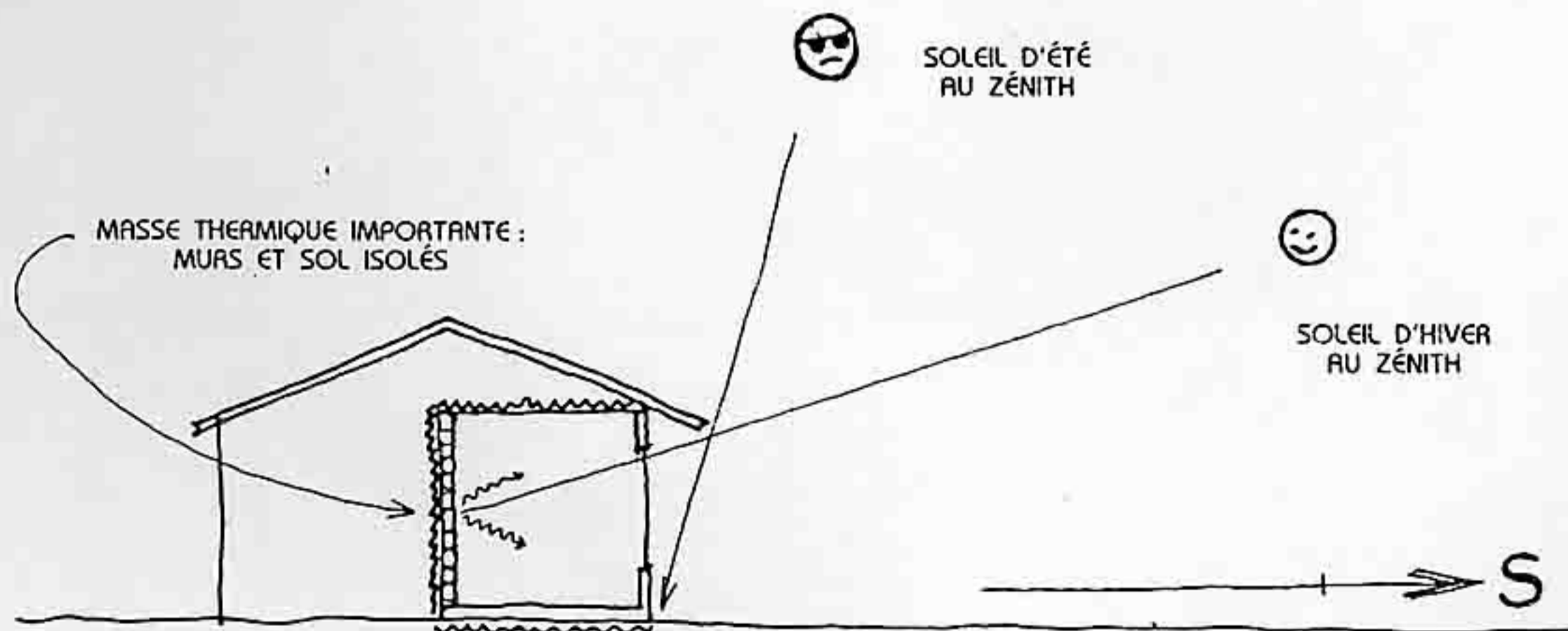
FIG. 6.21 : RELATIONS ENTRE SOLEIL, FENÊTRE ET AVANT-TOIT.
