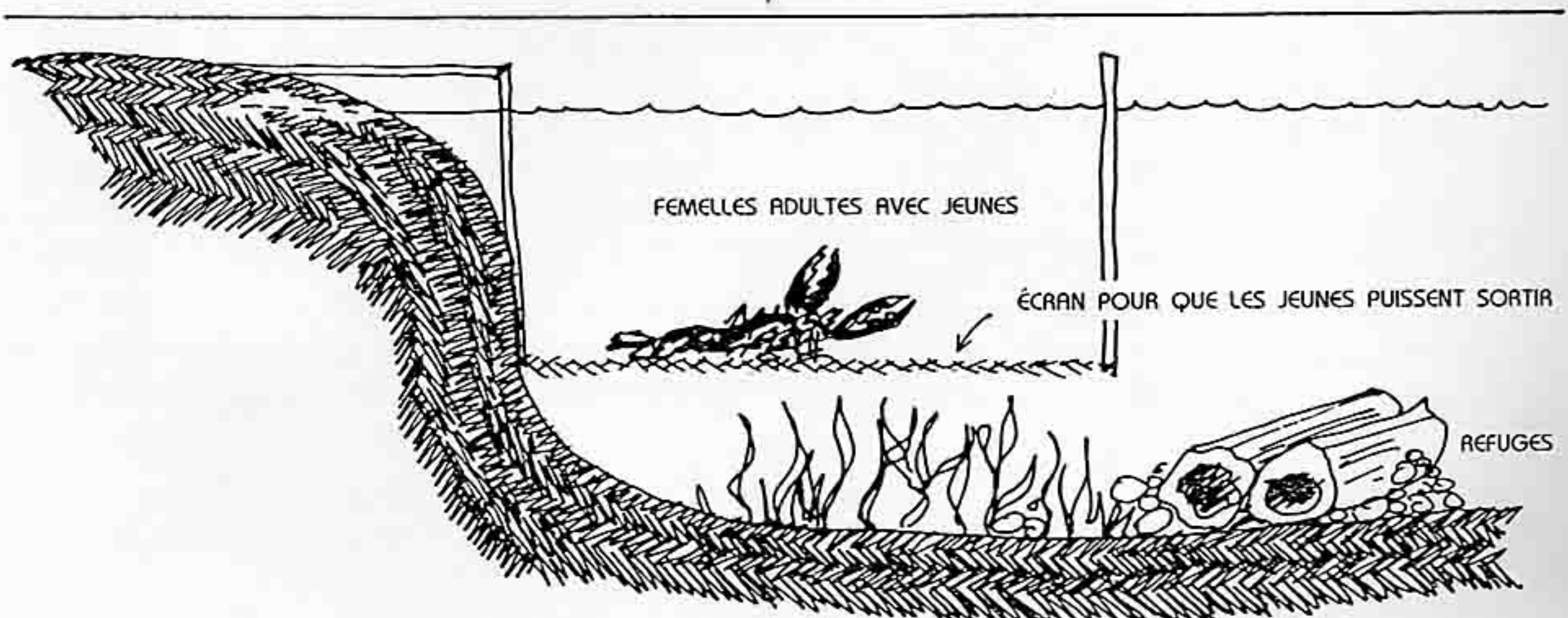
FIG. 7.19 : PANIER A FRAI POUR CRUSTACÉS D'EAU DOUCE PORTANT LEUR ŒUFS ET LEURS JEUNES SOUS LA QUEUE (ÉCREVISSÉS, HOMARDS).
