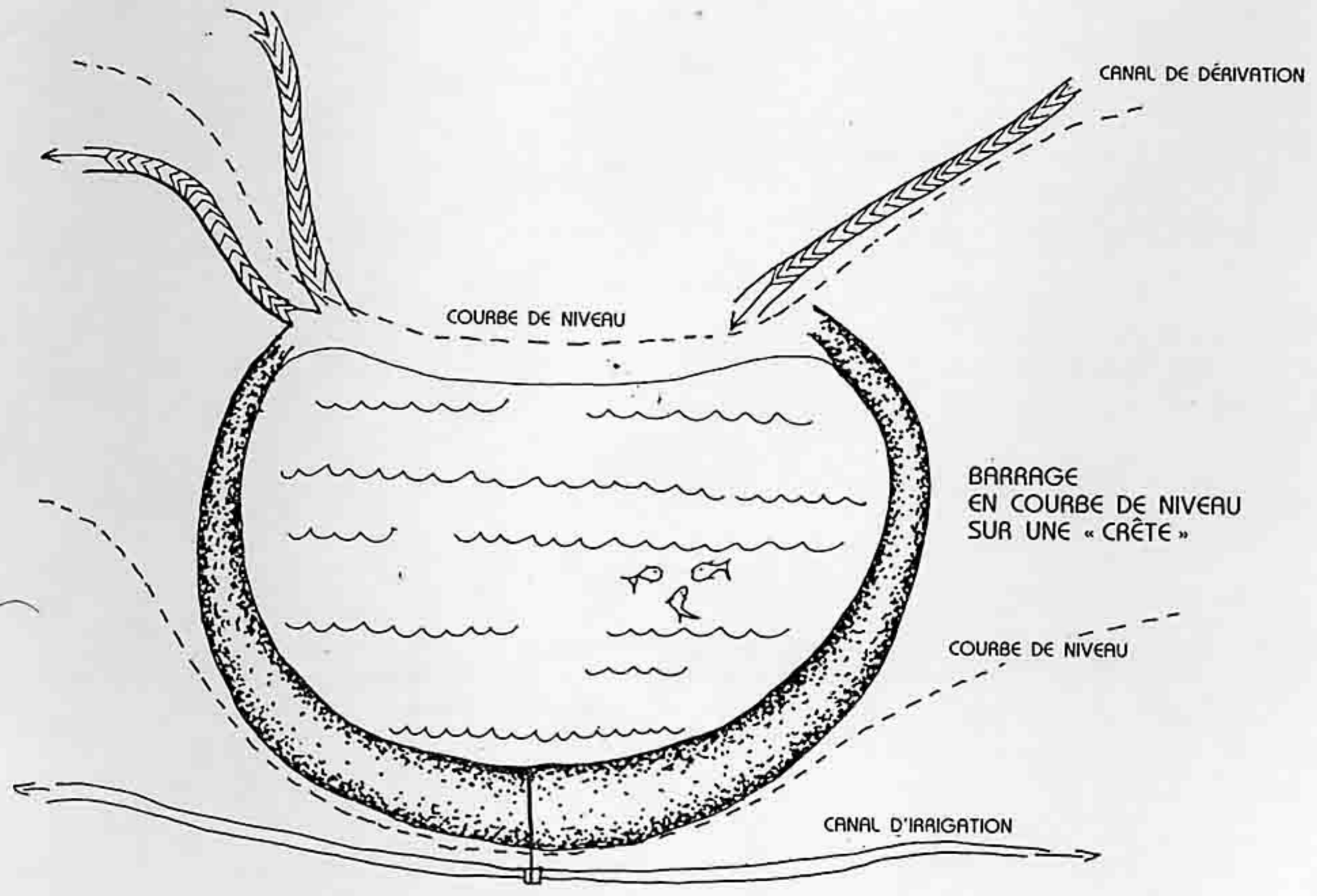
FIG. 7.4 : BARRAGES EN COURBES DE NIVEAU.
