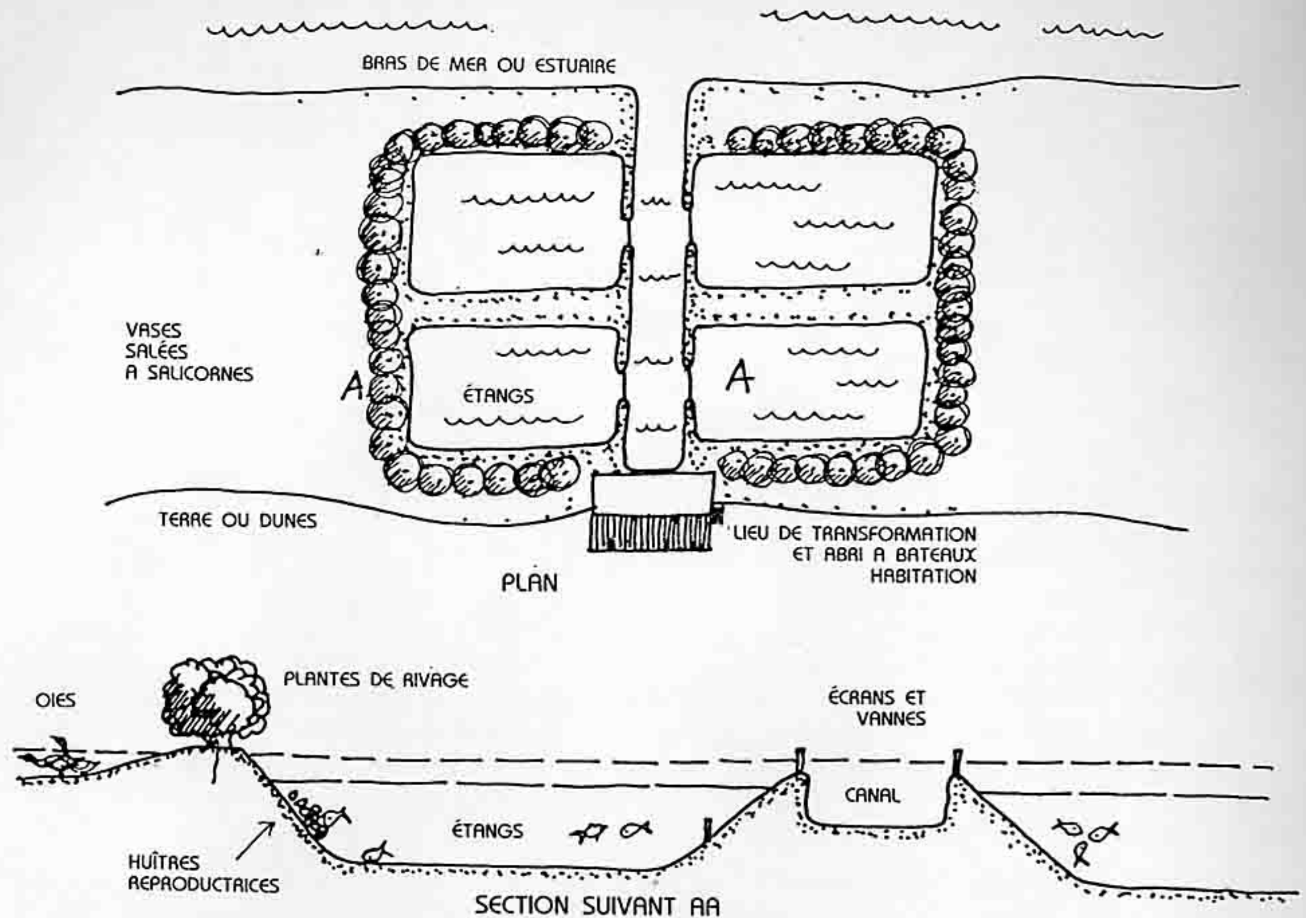
FIG. 7.24 : PLAN ET SECTION D'ÉTANGS À MARÉE.
