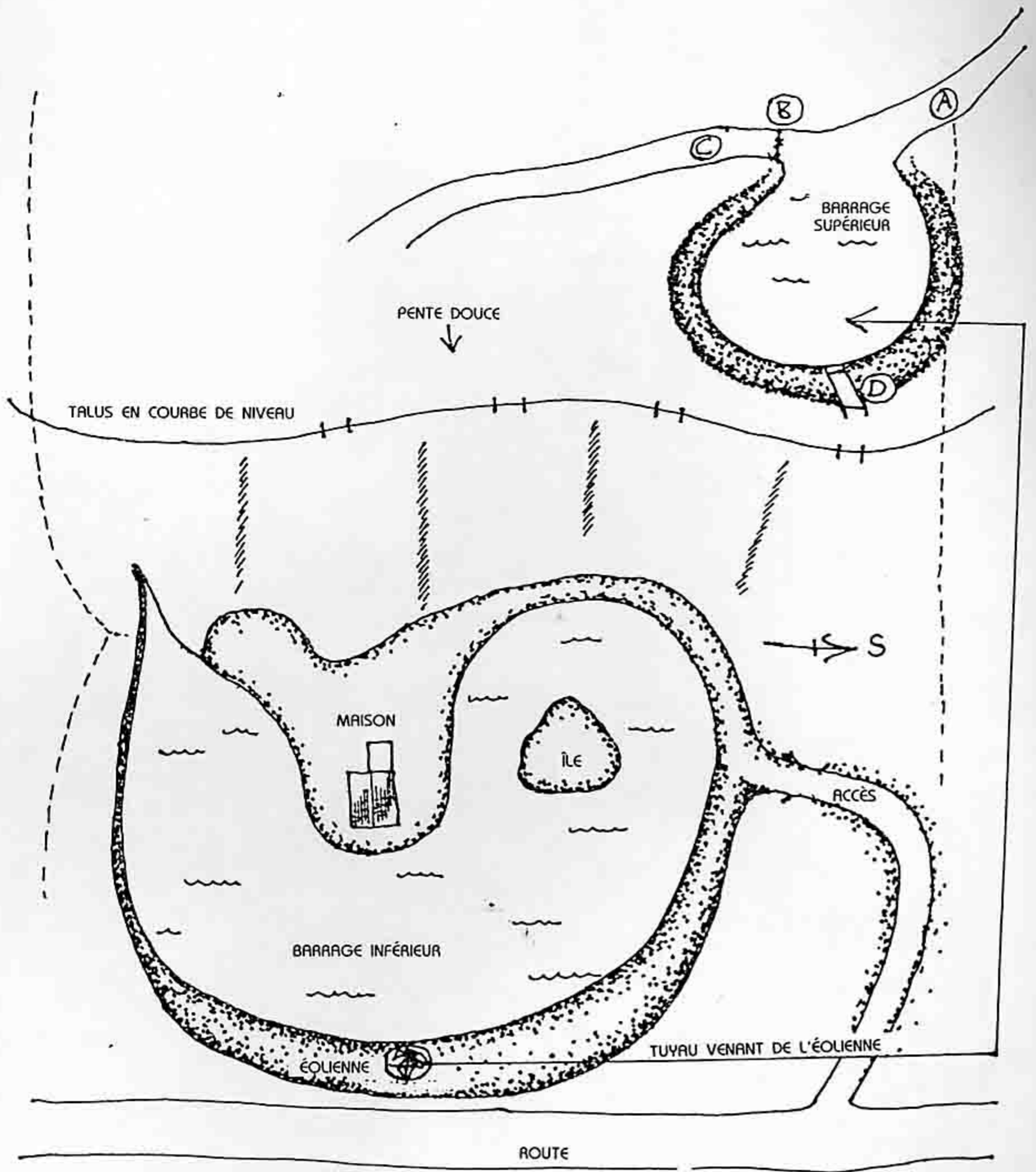
FIG. 7.13 : PLAN D'UN TERRAIN DE 2 HECTARES A DIGGER'S REST, VICTORIA. LA MAISON EST PROTÉGÉE DU FEU ET L'EAU EST CONTRÔLÉE SUR TOUTE LA SURFACE DU TERRAIN. CONCEPTION DE YEOMANS, GALL ET MOLLISON (VOIR DÉTAIL FIG. 7.14).
