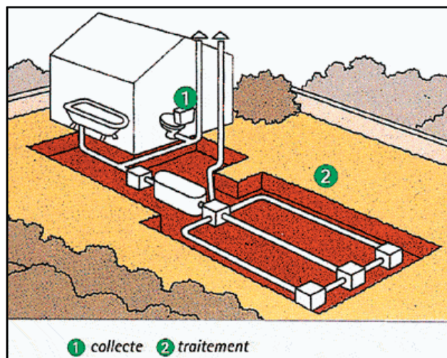
Assainissement individuel conventionnel
