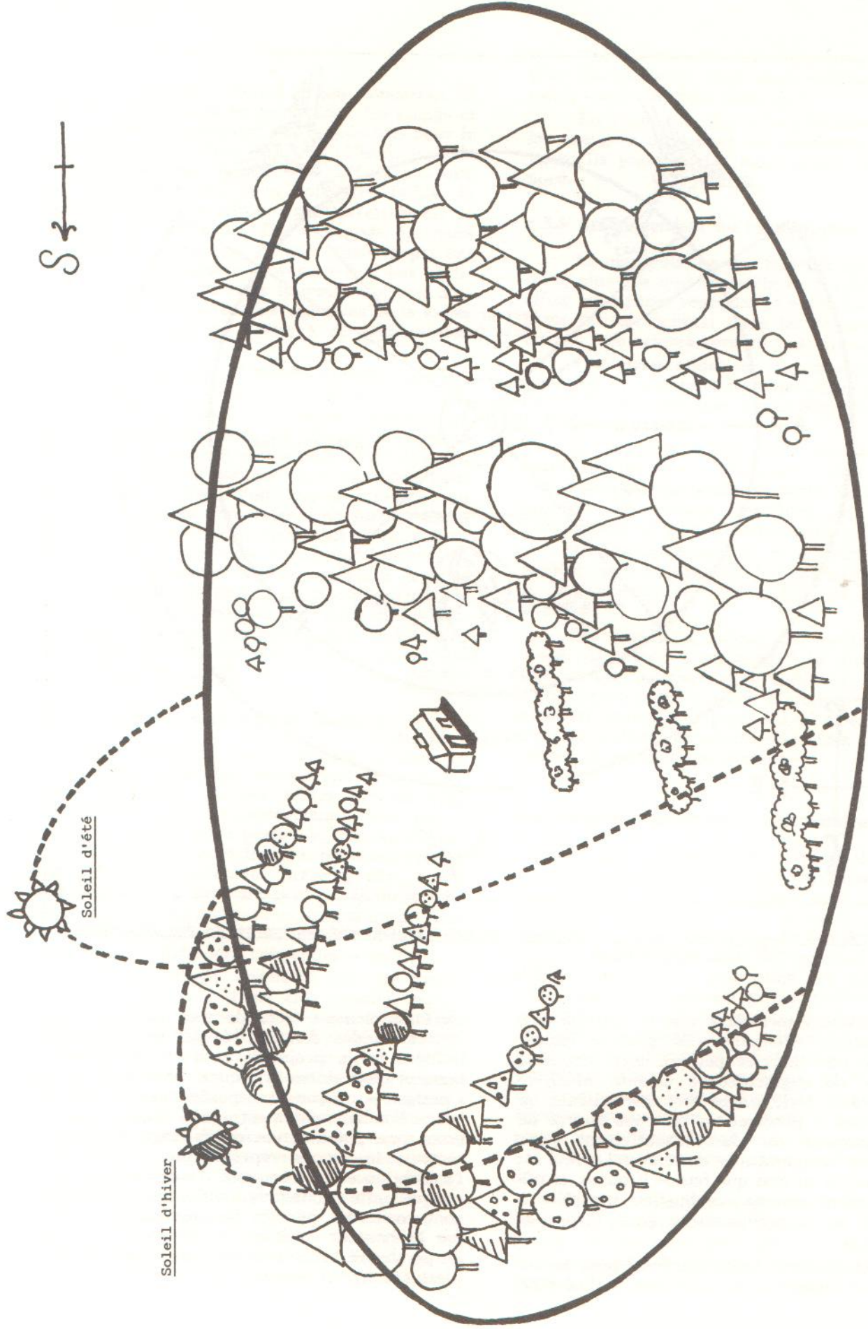
Figure 6.4.2 Les angles d'ensoleillement hivernal et estival commandent la hauteur des arbres dans la plantation. Les côtés exposés à l'ouest peuvent être fermés par des haies protégeant des vents froids
