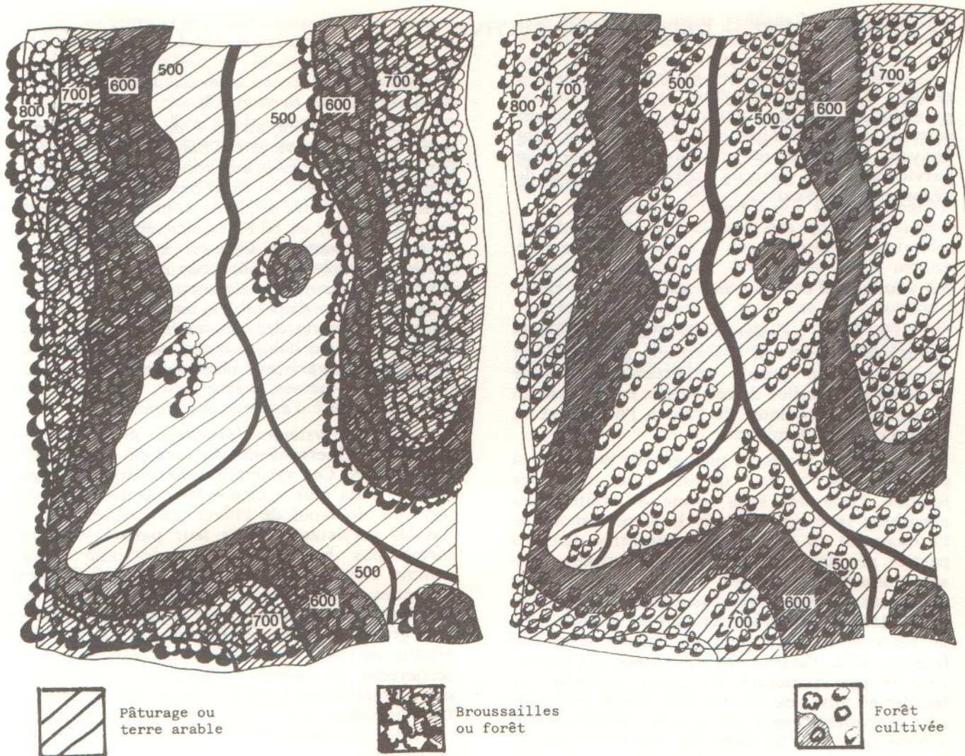
Figure 5.2.1 Disposition de la forêt (d'après Douglas)
