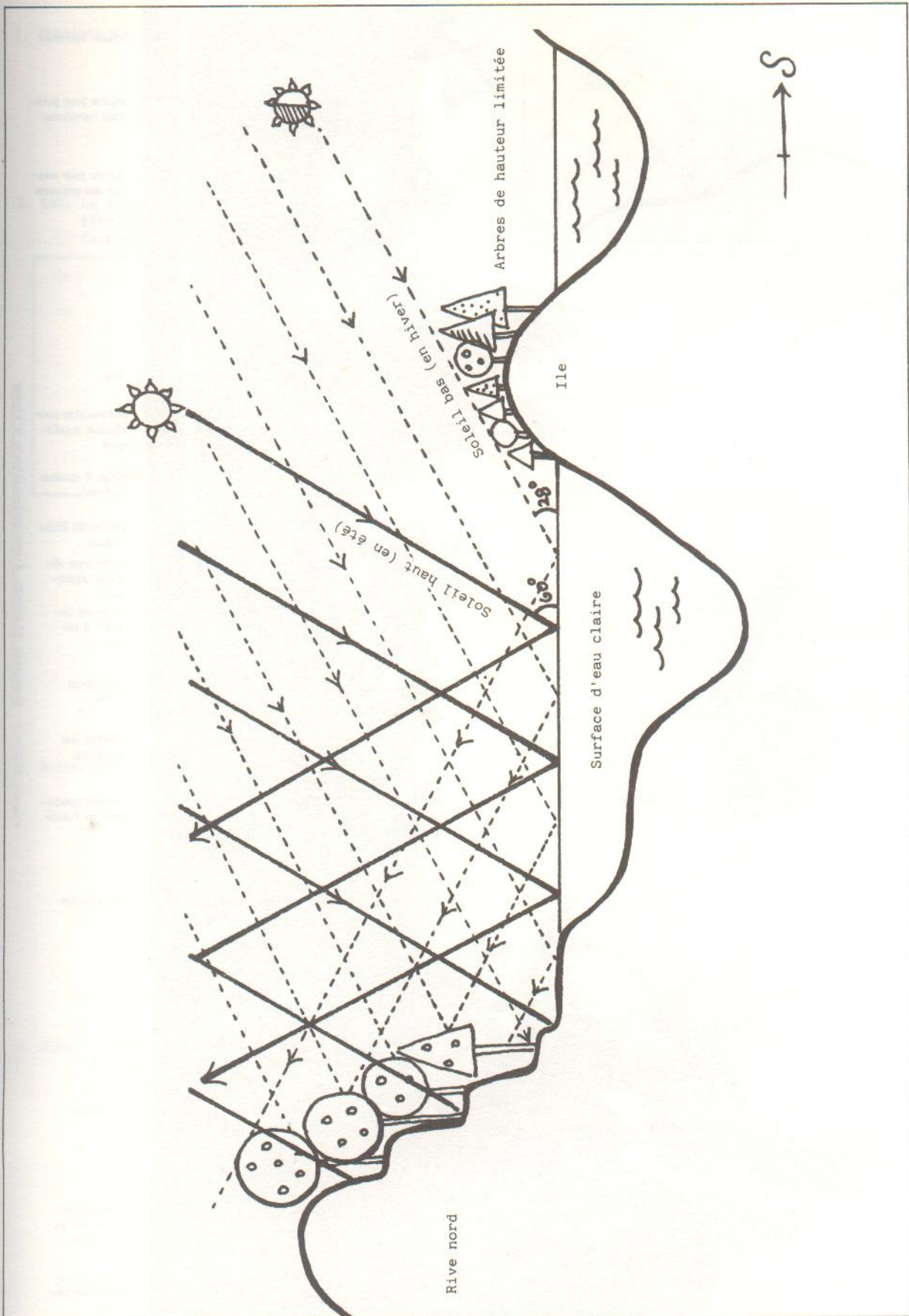
Figure 6.3.4.1_ Surface d'un étang utilisée comme réflecteur pour un ensoleillement à faible incidence angulaire. Les îles et les émergences fournissent des habitats spécialisés
