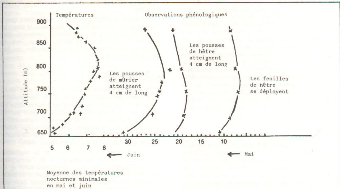
Figure 6.3.1.4 Relation étroite entre la température nocturne (à gauche) et la croissance des plantes sur le Grosse Arber (d'après Geiger, 31)
