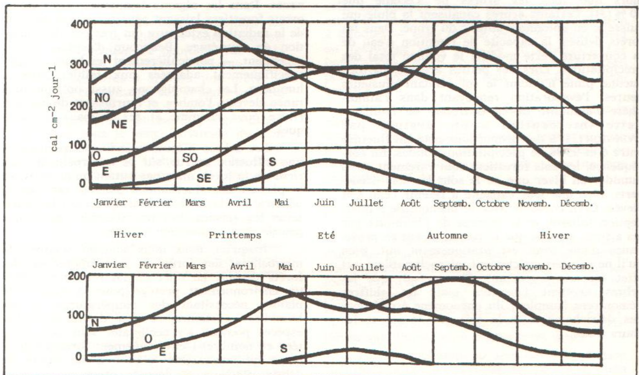
Figure 6.3.3.1 Totaux quotidiens de radiations solaires directes au niveau de lisières orientées différemment, par un jour ensoleillé (en haut), et par un jour ordinaire (en bas), pendant toute l'année. (Données originaires d'Europe centrale, Geiger, 31)
