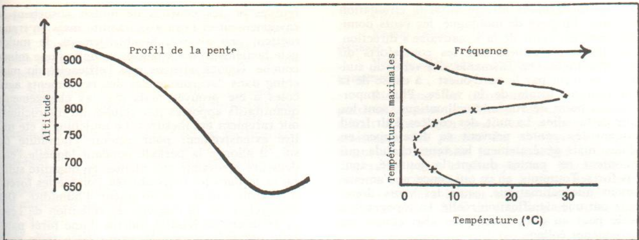
Figure 6.3.1.3 Localisation de la bande chaude sur les pentes du Grosse Arber au printemps (d'après Geiger, 31)
