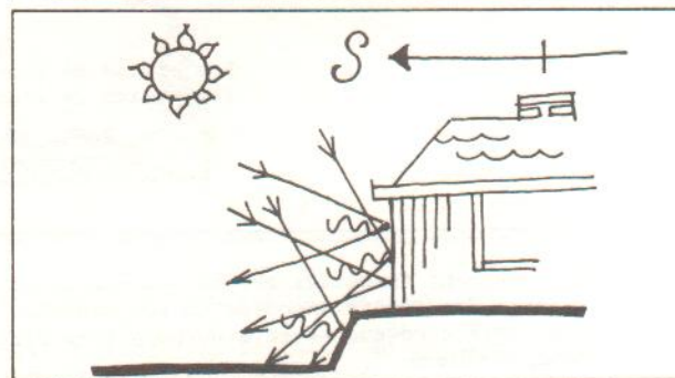
Figure 6.3.6.1 Éléments utiles pour l'accroissement du rayonnement et l'élévation de la température Les flèches indiquent l'incidence et le réfléchissement du soleil, les lignes sinuées la chaleur irradiée.
